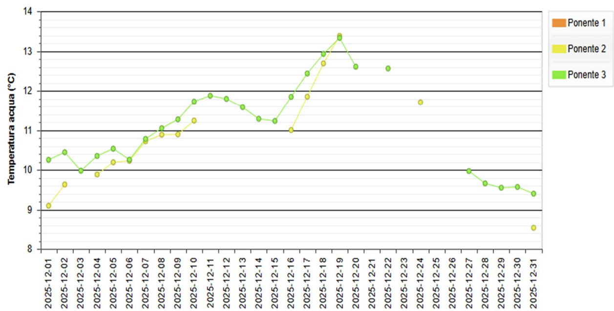
Figura 14 - Andamento medio giornaliero della Temperatura nella Laguna di Ponente.
