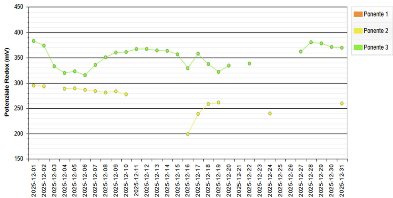
Figura 12 - Andamento medio giornaliero del Potenziale Redox nella Laguna di Ponente.
