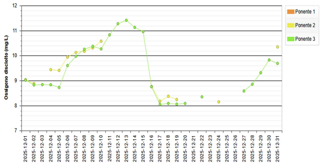
Figura 16 - Andamento medio giornaliero dell'Ossigeno disciolto nella Laguna di Ponente.
